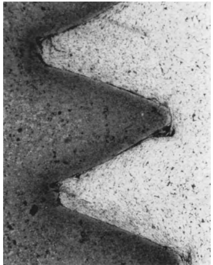
Spiralfarm® M4 x 16
